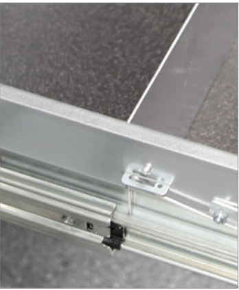
Arretierung der Schubladen im geöffneten Zustand
